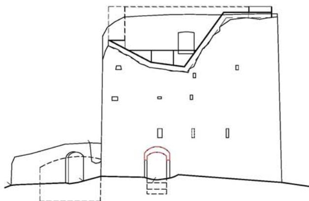
Façana nord-est
