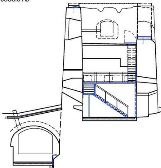
Secció AB
