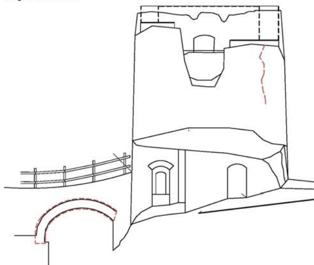
Secció CD
