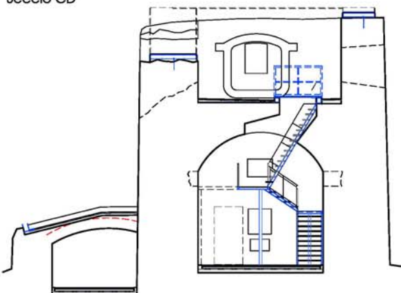
Secció CD
